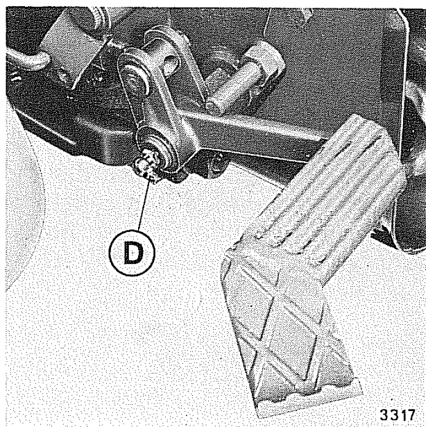
Fig. 21 - Punti d'ingrassaggio
