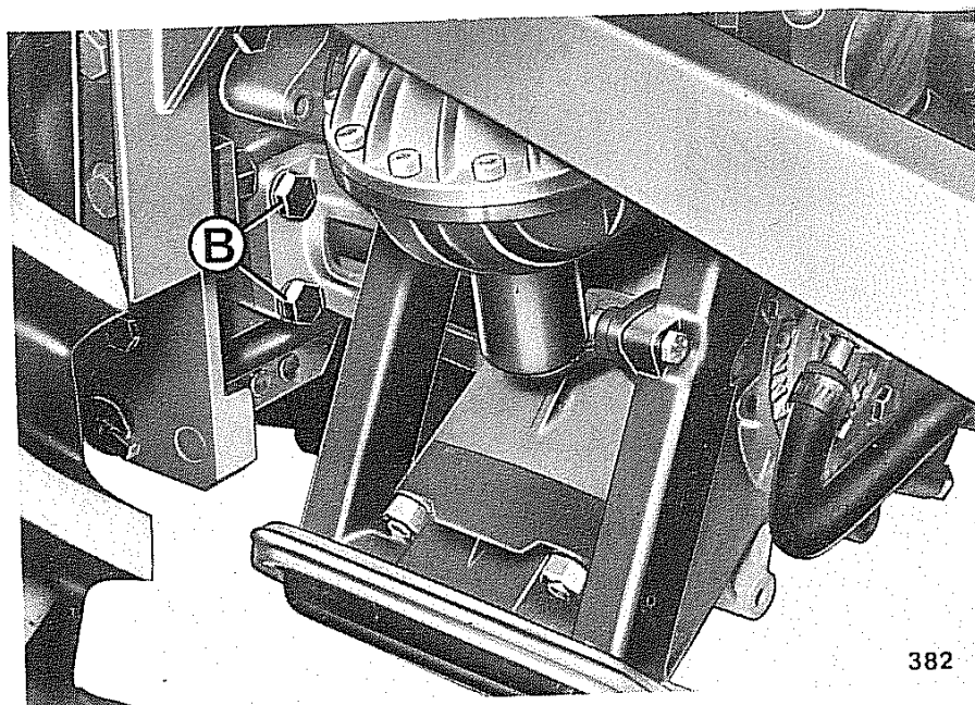
Fig. 103 - Attacco pompa
