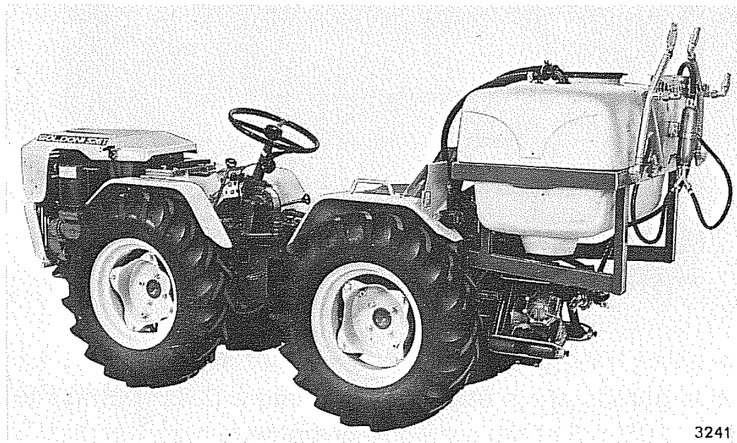
Fig. 100 - Gruppo irrorante
