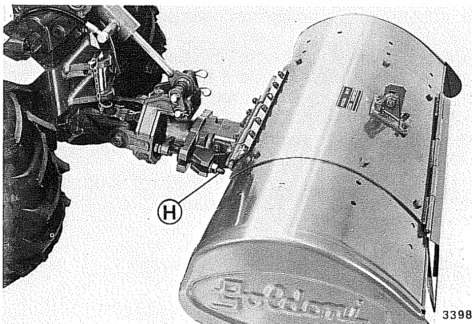
Fig. 45 - Fresa tipo "28"
