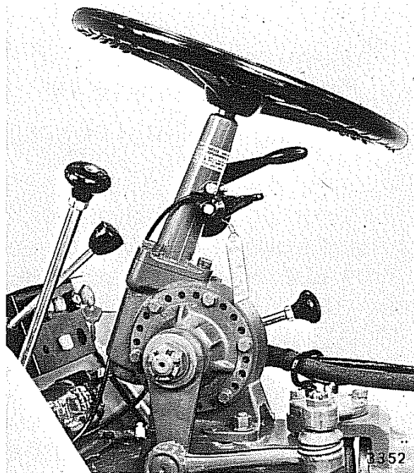
Fig. 16 - Sterzo meccanico
